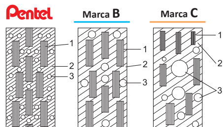
* 1. Grafite 2. Aglutinante 3. Poros (óleo)
